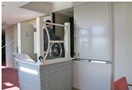
段差解消機
