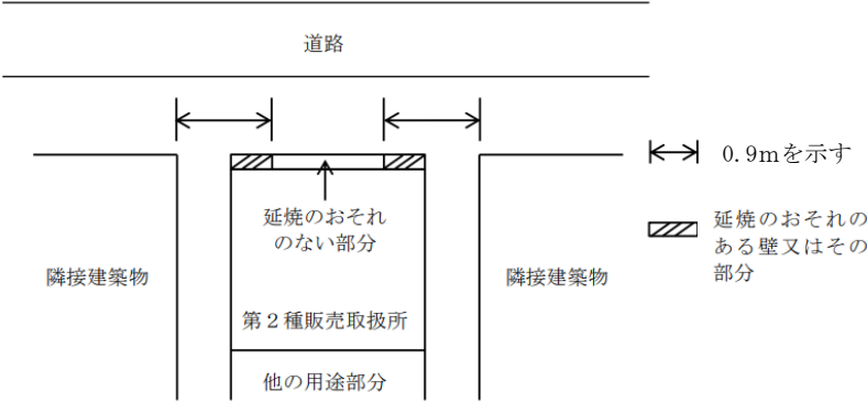
第 16-3 図 延焼のおそれのない部分の例
