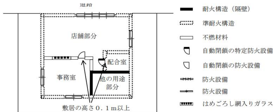
第 16-1 図 販売取扱所の設置例
