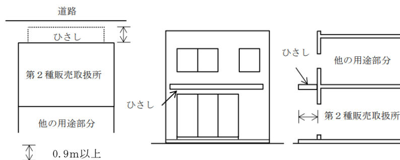
第 16-2 図 上階への延焼を防止するための措置例
