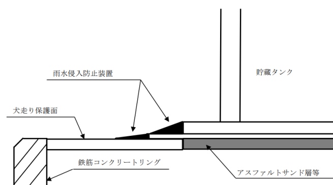
第 7-4 図 雨水侵入防止措置例 3
