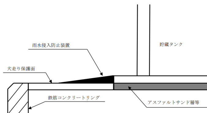
第7-2図 雨水浸入防止措置例1
