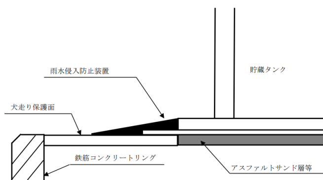
第 7-3 図 雨水侵入防止措置例 2
