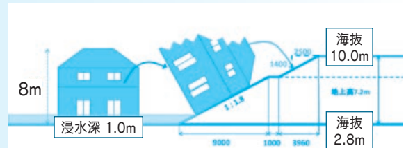
【図1】 津波による建物流出時の安全度評価
