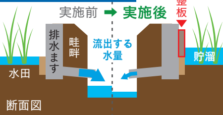
田んぼダムの仕組み
