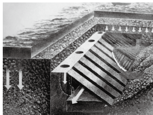
地下ダムの断面構造
