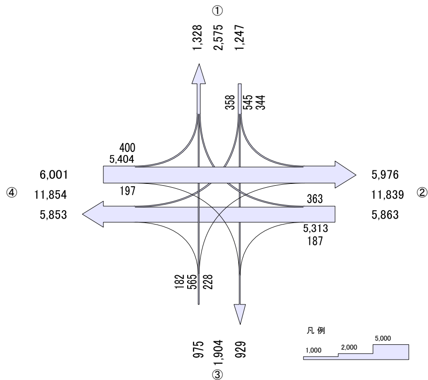
交通流帯図
