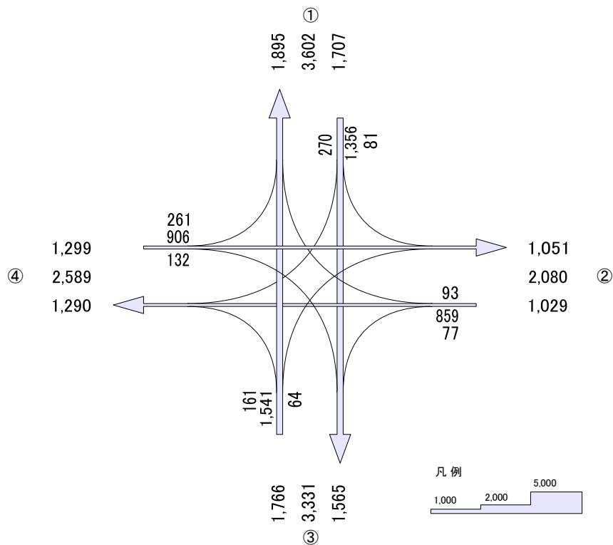
交通流帯図
