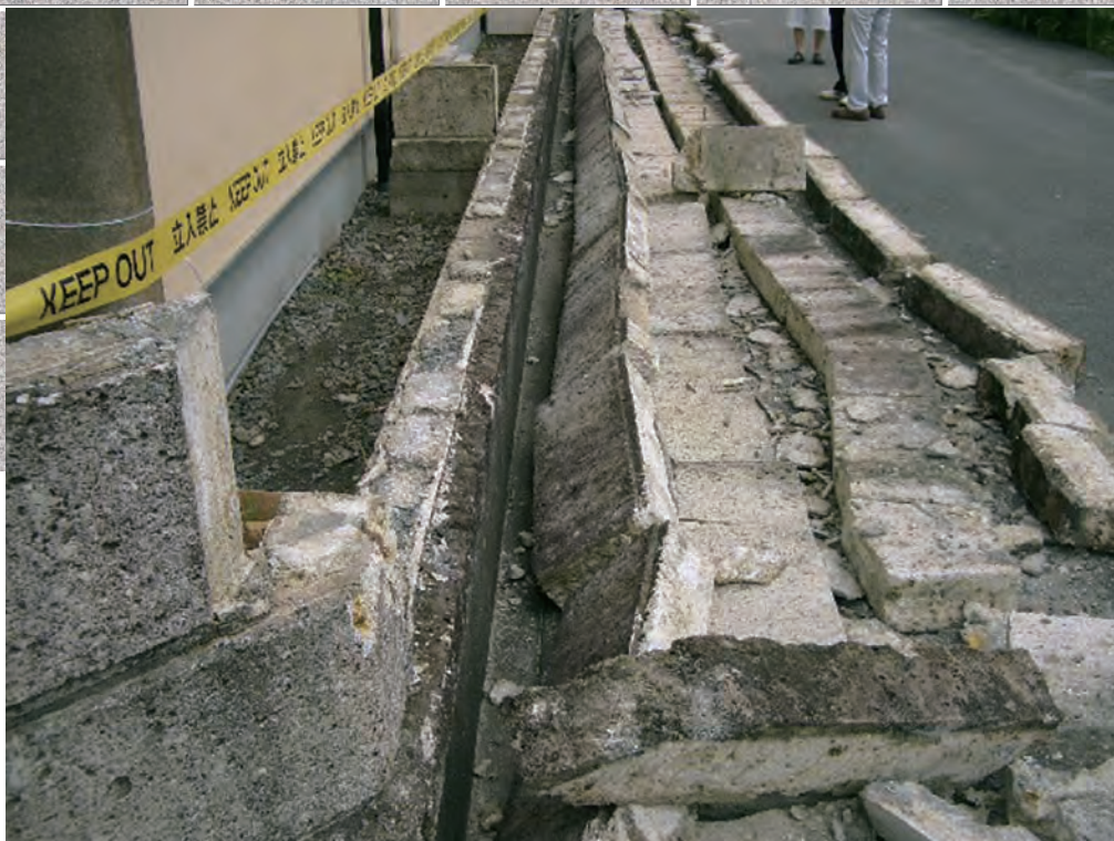
駿河湾を震源とする地震（平成23年8月1日発生）による大谷石堀の倒壊
