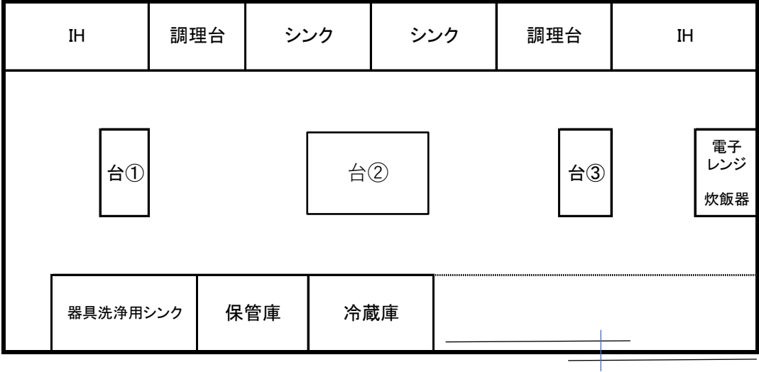
袋井学校給食センター食物アレルギー対応室 平面図
