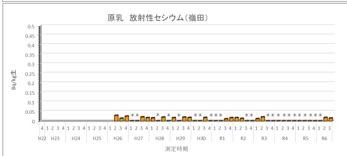
図3 原乳中の放射性セシウム濃度 (Cs-134 と Cs-137 の合計量) の経時的変化
