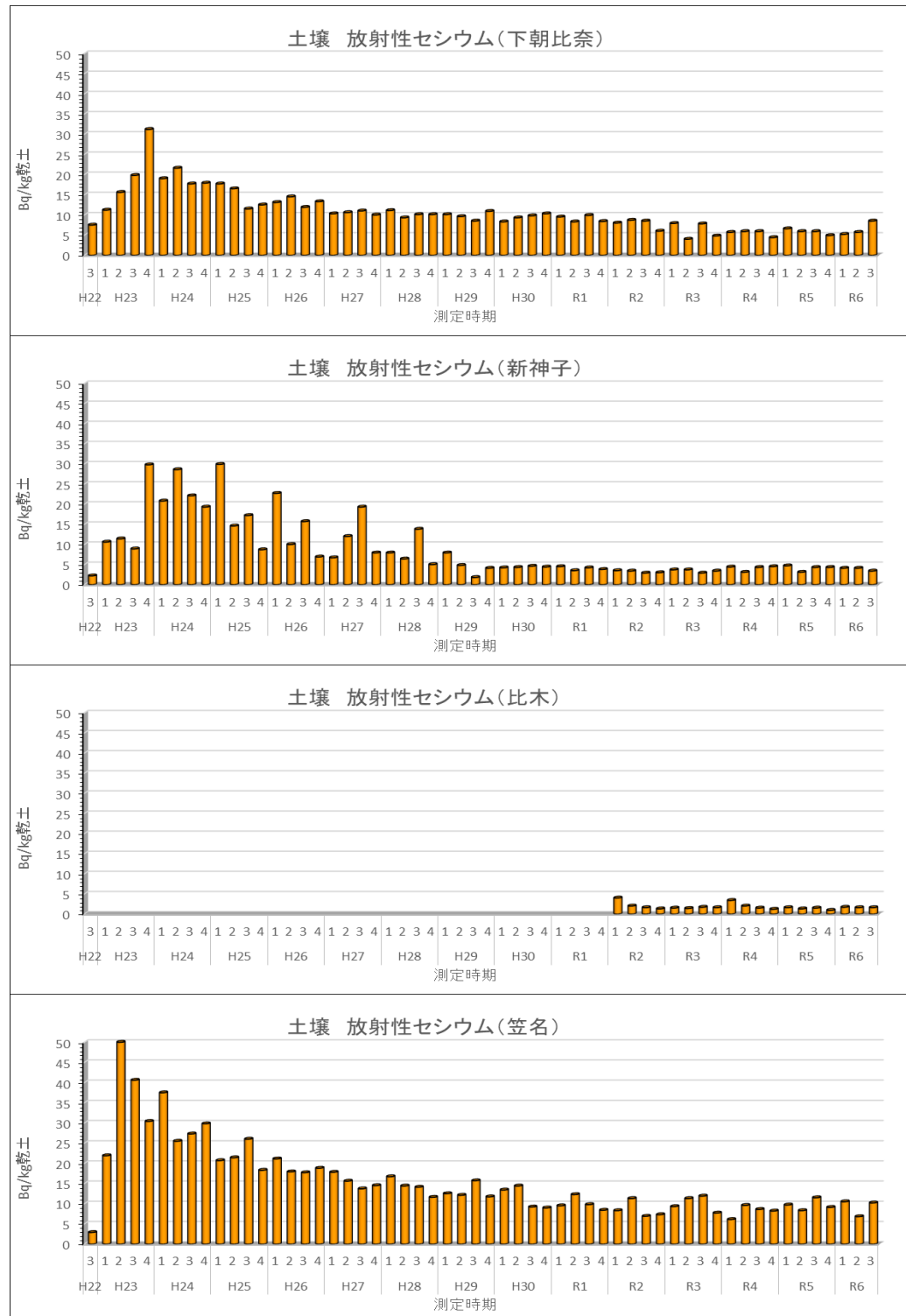
図1 土壤中の放射性セシウム濃度(Cs-134とCs-137の合計量)の経時的変化 注) 測定機関2者のうち、放射性セシウム濃度が高い値を採用している。
