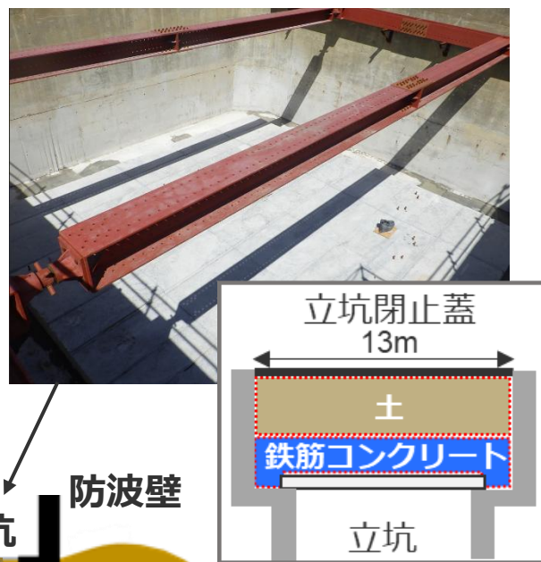
立坑閉止蓋 (現在の状況 (2026.6時点) )
