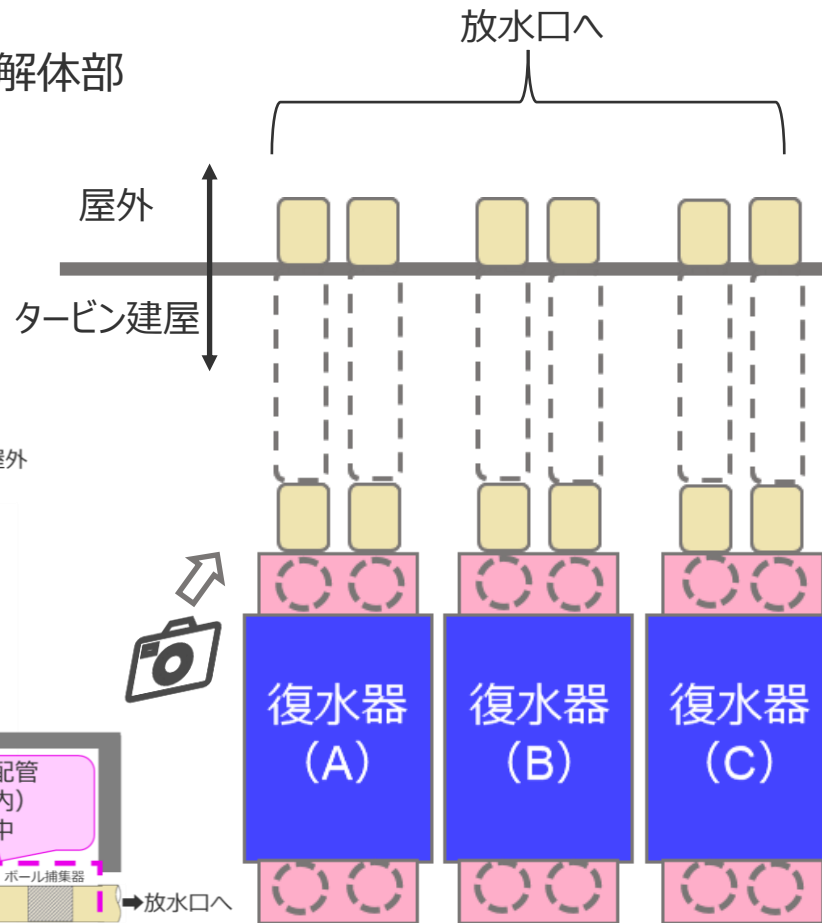
<平面図>
